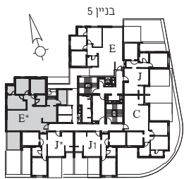
תוכנית קומות 2-4
